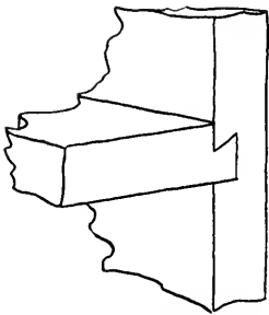
DOVE-TAIL DADO
